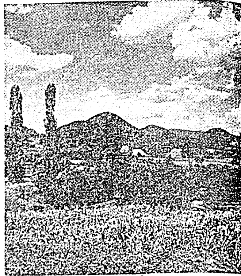
Conurile vulcanice la Cămarăna în lanțul nordic al Carpaților Orientali.
