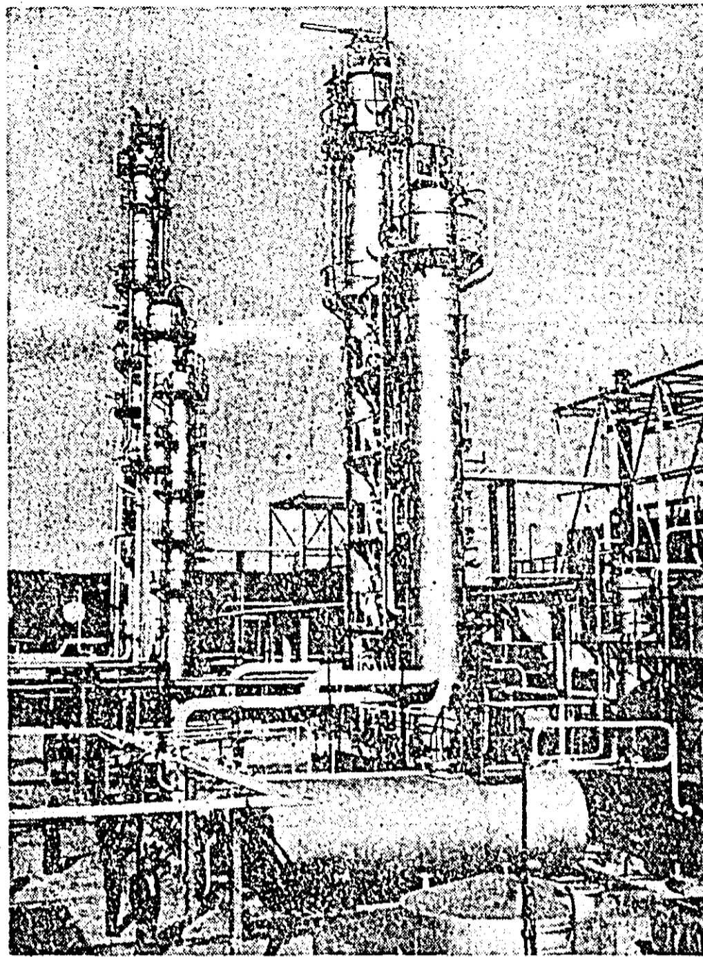
Un nou obiectiv industrial: Rafinăria 10 Onești — instalația de absorbție și fracționare a gazelor.
