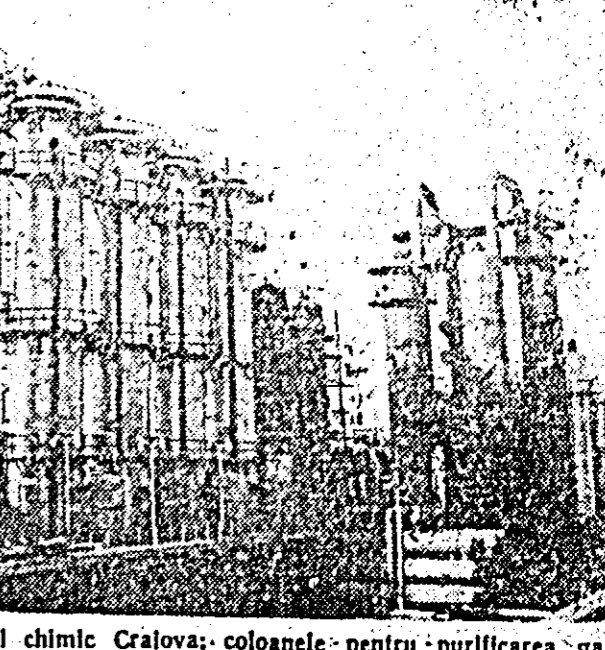
Combinatul chimic Craiova: coloanele pentru purificarea gazului de sinteză ale fabricii de amoniac.
