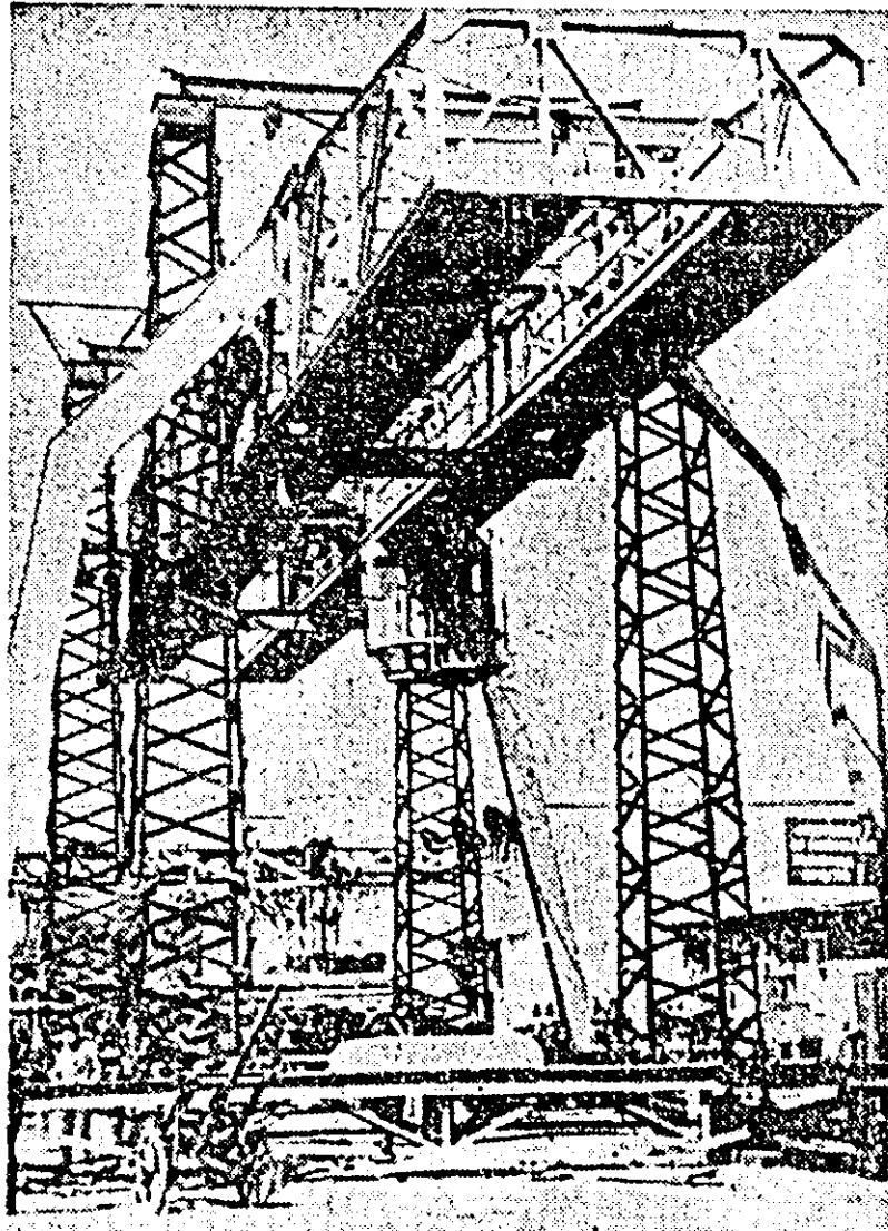
La sectorul I al Uzinelor de vagoane se lucrează la montarea unei macarale de 5 tone care va ușura mult transportul materialelor.
