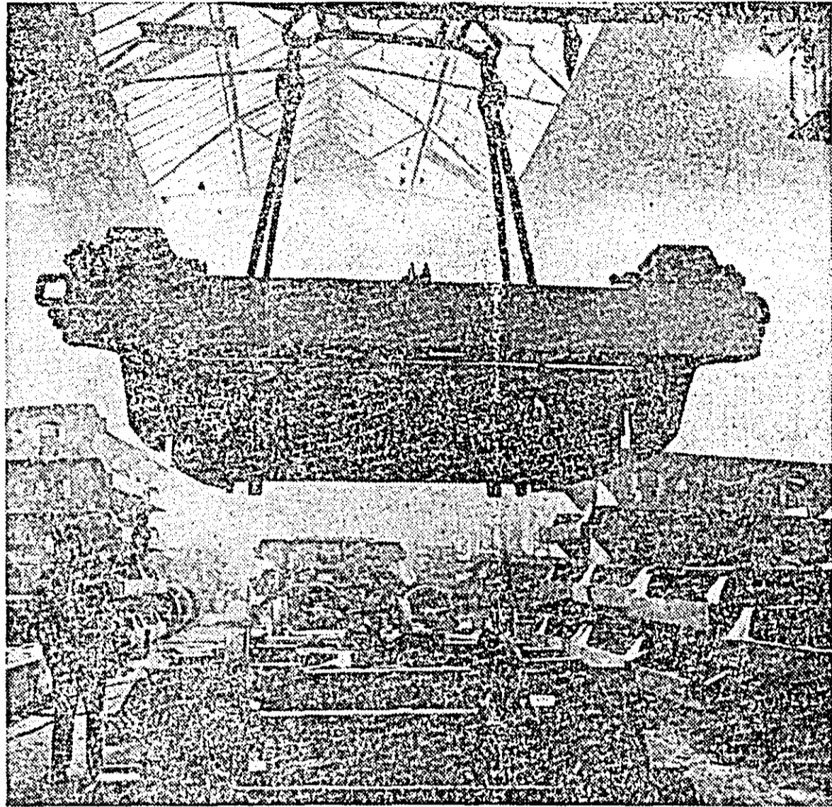
Uzinele de vagoane. Aspect din secția boghului
