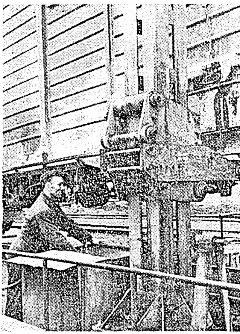
Atelierul de zonă CFR Curtici. Dispozitivul pentru ridicarea vagoanelor încărcate permite repararea operativă a defecțiunilor vite, nemaifiind necesară transbordarea încărcăturii vagoanelor. Autorul dispozitivului e lăcătușul montator Traian Deac.
