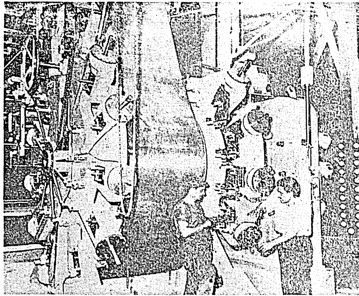
Secțiile uzinelor „30 Decembrie” sînt dotate continuu cu utilaje moderne, care ajută colectivului să obțină producții sporite. Iată un aspect din timpul montării unei noi mașini de imprimat de mare capacitate. Una din caracteristicile ei tehnice, este aceea că se poate imprima în zece culori.
