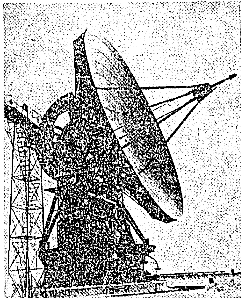
Radiotelescop parabolic PT-22 realizat în Uniunea Sovietică. Ogînda avînd un diametru de 22 m și o distanță focală de 9,5 m se rotește în planele orizontală și verticală. Telescopul permite să se efectueze cercetări în gama undelor centimetrice și a undelor mai mici de 1 cm.
