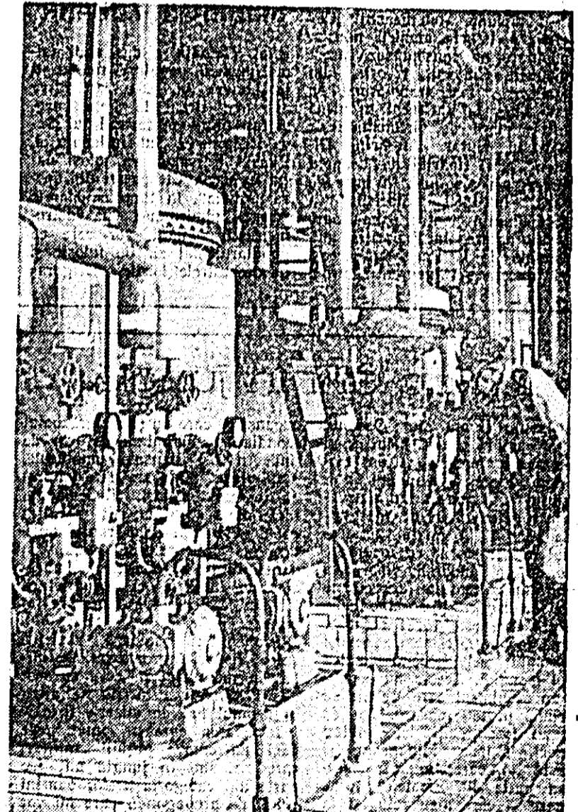
R. P. CHINEZA. — Secția de alcool polivinilic de la Fabrica de vinlon, cea dintîi fabrică de acest gen din R. P. Chineza, a intrat recent în producție. Proiectarea, fabricarea și instalarea întregului utilaj al fabricii, este executat de muncitorii și inginerii chinezi. ÎN FOTO: Aspect de muncă din secția alcool polivinilic recent intrată în producție.
