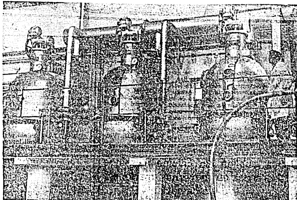
Utilajele moderne cu care este înzestrată fabrica Refacerea asigură realizarea unor conserve de bună calitate.
