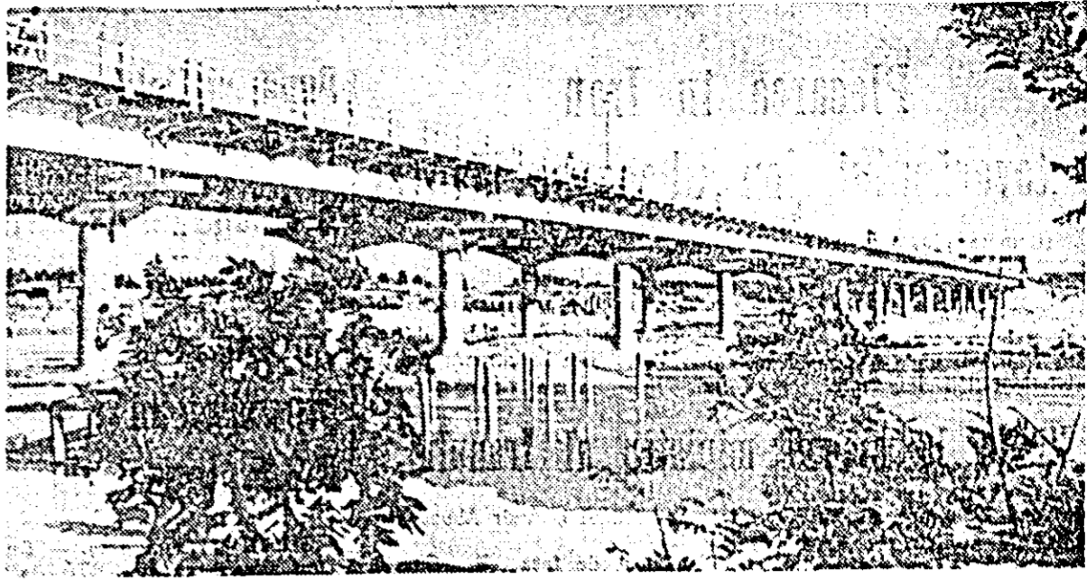
În provincia Honan, R. P. Chineză în apropierea orașului Nanyang, s-a construit nu de mult un pod la care s-a aplicat o nouă metodă de construcție. Podul cu o lungime de peste 400 m, se sprijină pe 19 stâlpi de beton și a fost construit numai în 40 zile.
