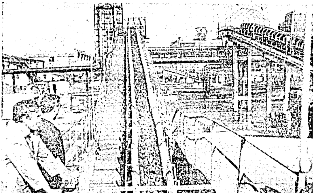
La întreprinderea de Industrializare a sticlei de zahăr, rampa de încărcare-des- cărcare asigură integral cantitatea de materie primă necesară funcționării instalațiilor la parametri proiectați — cite 4000 tone rădăcină în 24 ore.
