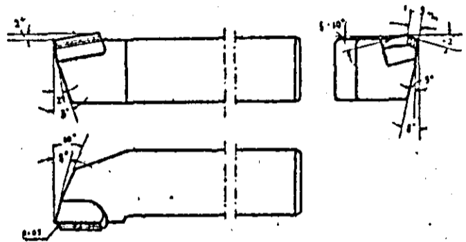
Cuștil de strung tip Bortkievici
