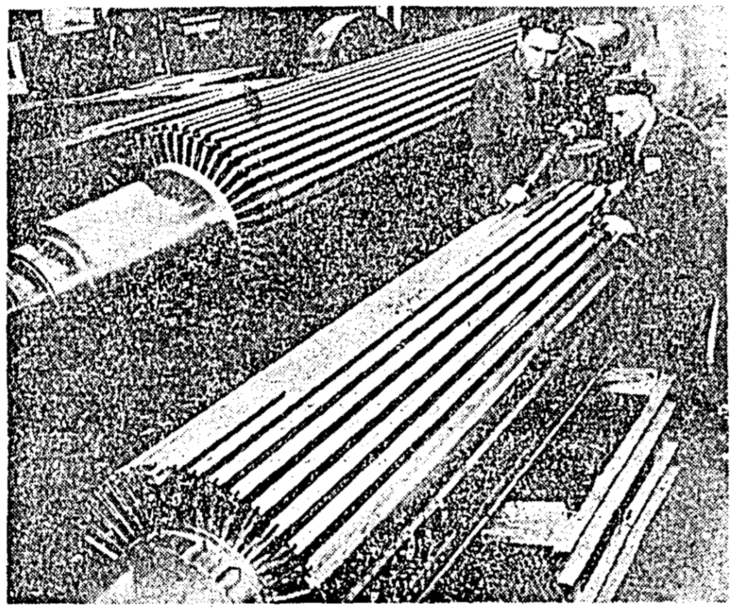
Uzinele de uzină greu „Electrotehmag” din Harkov (U.R.S.S.) produc generatoarele gigantice „TGV-300” destinate șantierelor de construcții. Pentru construirea lor se folosește material izolant termoreactiv care permite mărirea capacității de producție a generatoarelor pînă la 330 mil kilowați.
