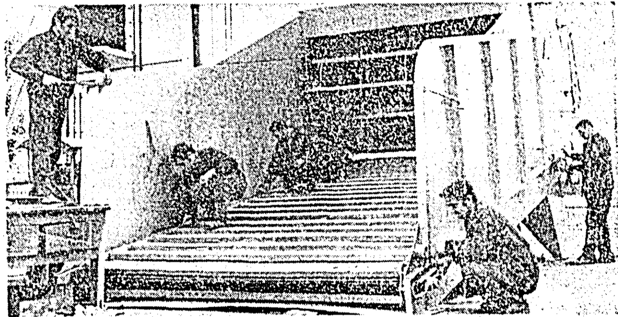
În discuție un nou și important produs al Uzinei de reparații — alimentatorul dozator pentru în-silozarea păloșelor.
