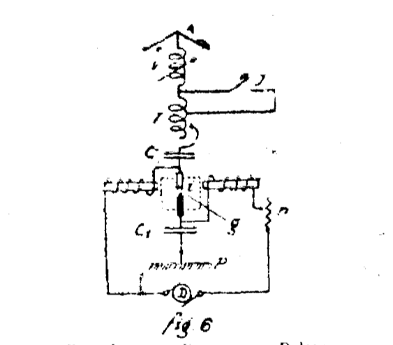
Post de transmitere cu arc Poulsen.
