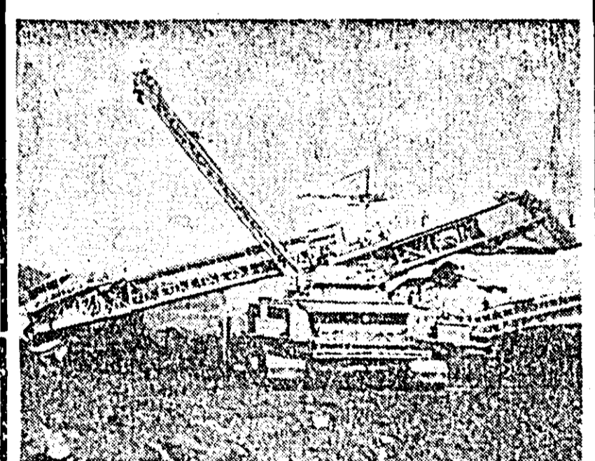
R. S. CEHOSLOVACA - Aspect de la mina de cărbuni Vintirov, unde au fost mecanizate aproape în întregime lucrările de extracție a cărbunului. ÎN FOTO: Excavatorul „K-300” de la mina Vintirov.
