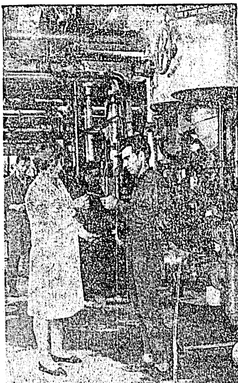
Usina electrică. La stația de tratare și demineralizare a apei — care va fi dată în funcțiune peste puțină vreme — se execută ultimele lucrări la montarea aparatelor de măsură și control. IN FOTOGRAFIE: exigență față de calitate, ing. Sofia Ghiță și tehnicianul Gh. Păcurar urmăresc mersul lucrărilor.
