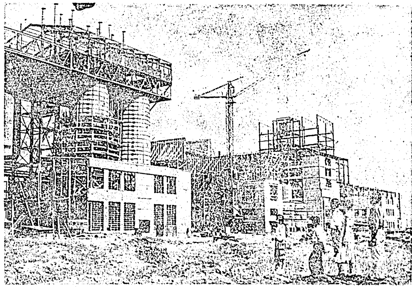
Lucrările de construcție a uzinei de produse sodice din Govora continuă. La secția var se lucrează la clădirea reactorului și la cupola deconcentrului de saramură care are o deschidere de 20 m în diametru.
