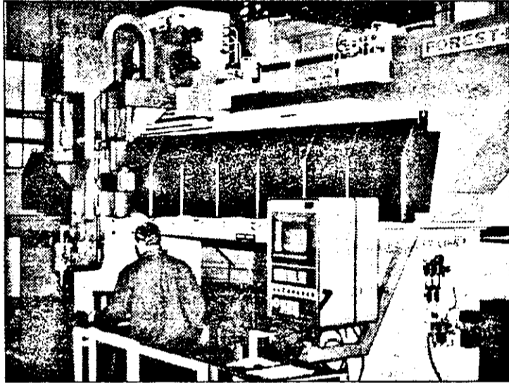
Cu această modernă mașină de frezat în coordonate sunt prelucrate reperi ce intră în componența boghiurilor cu care sunt echipate vagoanele de mare viteză (200 km/h) de tip Coraille. Mașina este amplasată într-o mică hală a secției Boghiuri (sectorul I - ASTRA), unde i s-au creat condiții speciale pentru a funcționa la parametri optimi.
