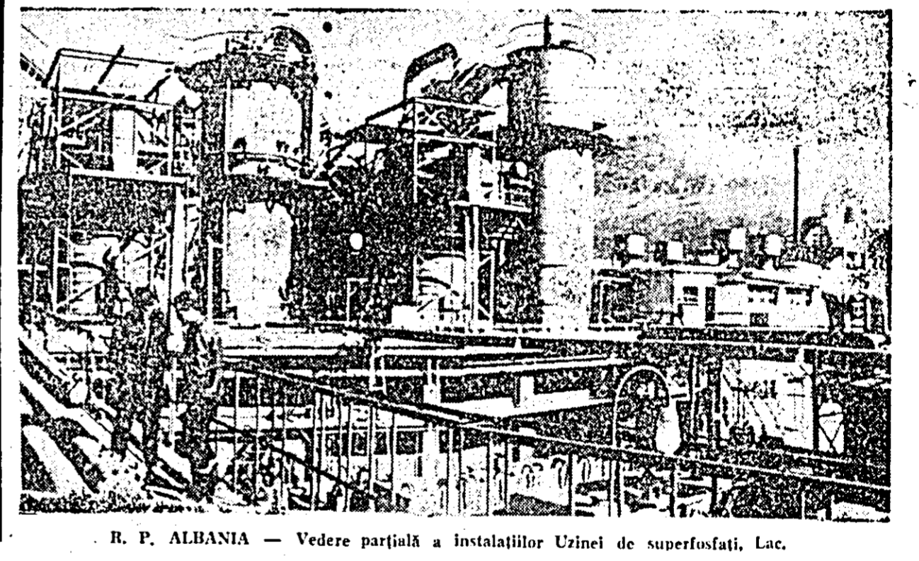
R. P. ALBANIA — Vedere parțială a instalațiilor Uzinei de superfosfați, Lac.
