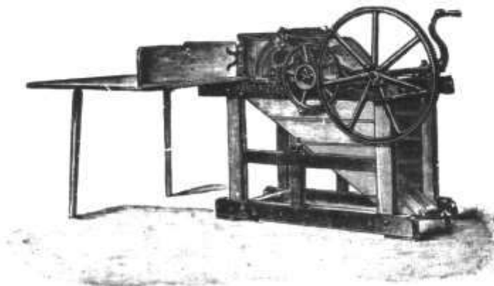
Batoza pentru acționarea manuală, având toba cu cuie (Rieger)
