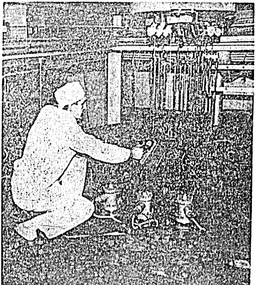
U.R.S.S. — Constructorii sovietici au creat o centrală electrică atomică care se poate transporta. Ea este compusă din blocuri separate care au o greutate de 4-22 tone fiecare. Capacitatea de producție a unei astfel de centrale este de 750 kilovați. IN CLIȘEU: verificarea radiațiilor.
