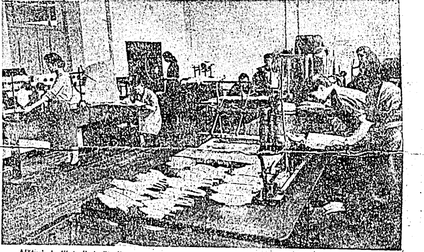
Alături de filatorii, țesătorii sau muncitorii sectorului țesuturilor, de la uzinele „30 Decembrie”, o activitate rodnică desfășoară și muncitorii și tehnicienii laboratorului fizico-mecanic. Aici ei fac analiza pentru determinarea calității materialelor prime, a firelor și țesăturilor, pentru ca ele să se încadreze în prevederile standardurilor în vigoare. Astfel, prin acest control se poate urmări calitatea produselor, contribuind în mod continuu la îmbunătățirea ei. IN CLÎȘEU: aspect din laborator, în timpul lucrului.
