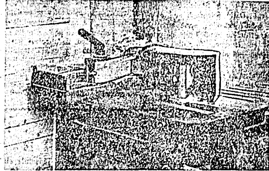
Această mașină simplă, inițiată de tov. Ștefan Vigh, a fost pusă în funcțiune în sectorul calapoade al fabricii de încălțăminte „Liberatea”. Cu ajutorul ei se frezează fața tocului, operație ce se execută înainte manual.
