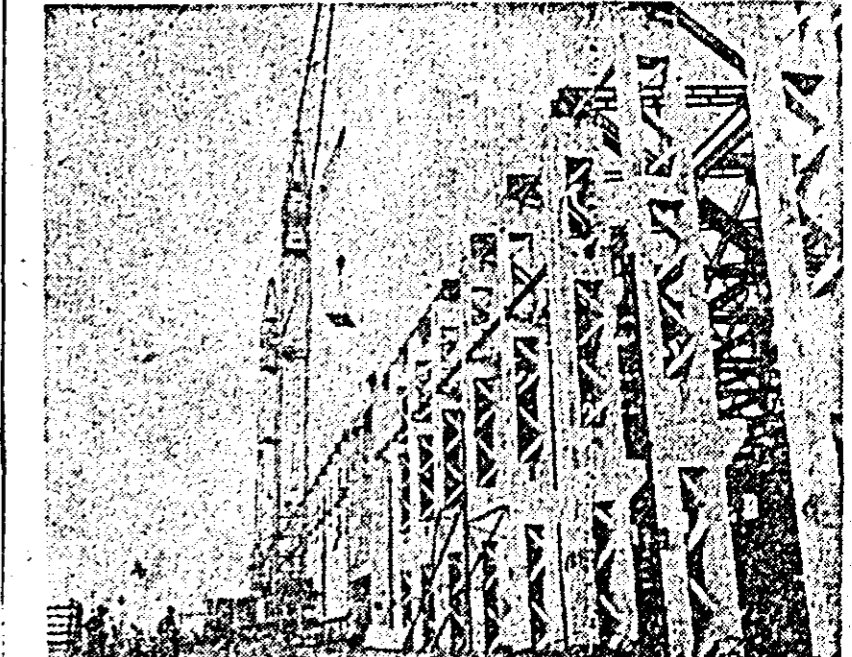
Vedere parțială a unei dintre cele două hale de electroliză (fiecăre avînd o lungime de 540 m) de la Uzina de aluminiu Slatina.
