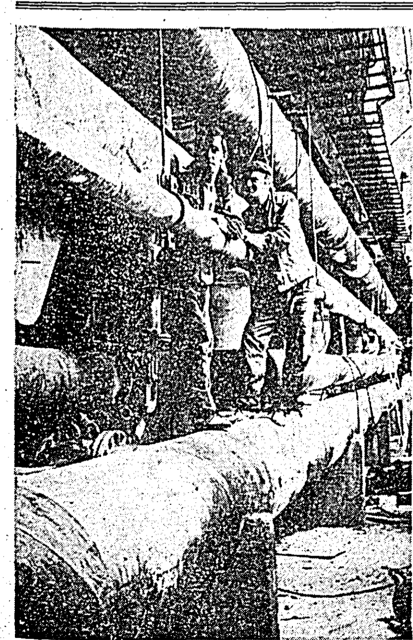
Se instalează conductele la noua uzină de apă a municipiului. Foto: M. CANCIU
