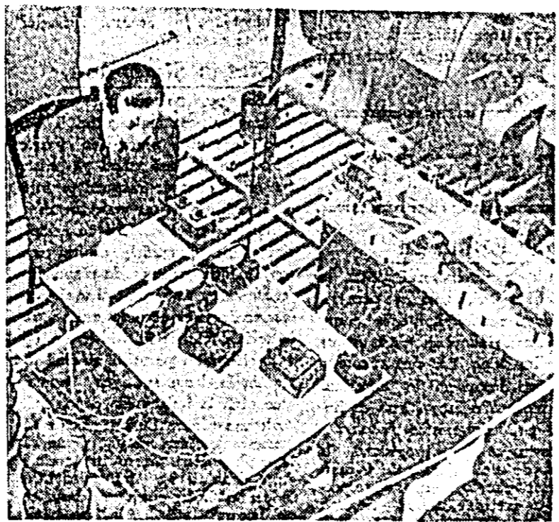
În laboratorul de mașini și transformatoare al Institutului de cercetări și proiectări pentru industria electrotehnică din București. Fotografia a fost luată în momentul executării unor încercări de încălzire la prototipul de transformator cu înfășurări din conductori de aluminiu izolați cu email.
