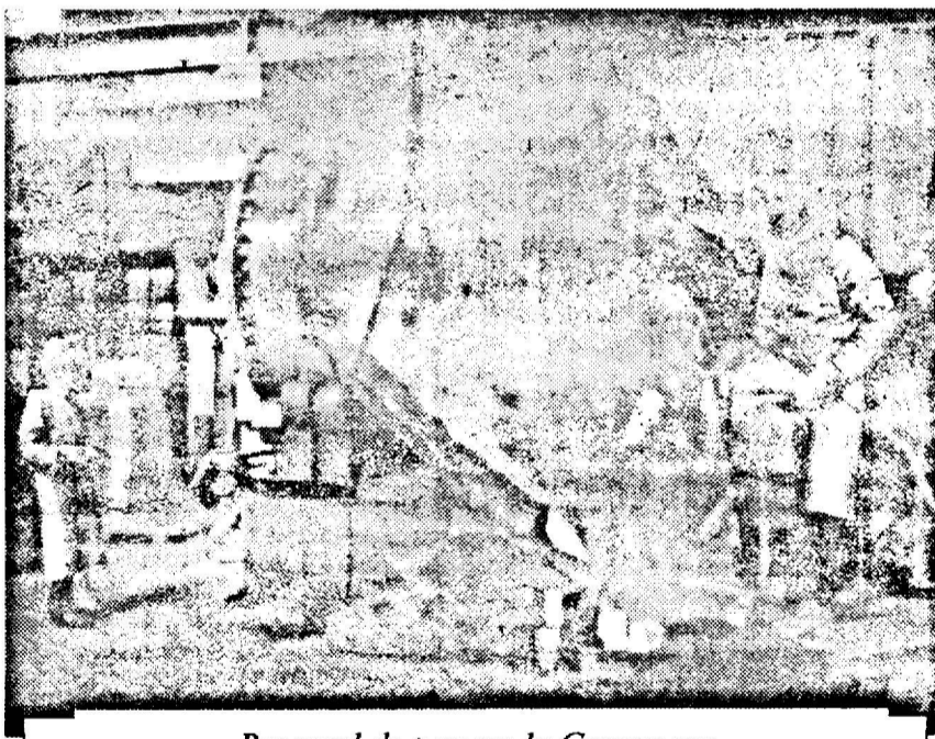
Procesul de turnare la Grossmayer
