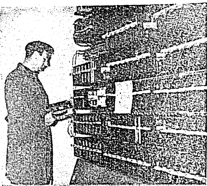
Sectorul centralizat electro-dinamic din stația CFR Arad. Funcționarea ireproșabilă a aparatului este urmărirea și verificarea cu toată exigența. Foto: DRAJA PAUL.
