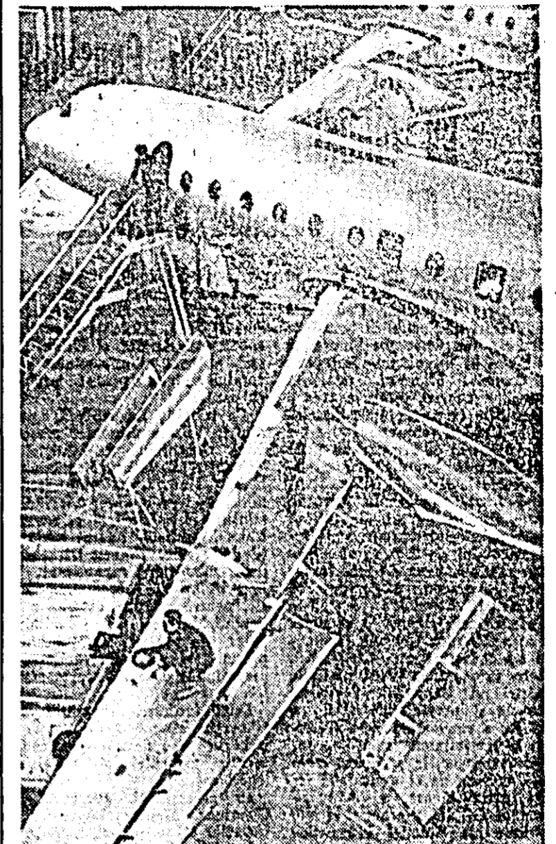
La uzina constructoare de avioane din Harkov (URSS) se produc acum avioane de pasageri cu reacție „TU-134” cu 72 de locuri. În diferitele condiții ale zborului se menține o anumită presiune, temperatură și umiditate. Viteza de croazieră este de 850-920 km pe oră, încălzirea comercială — 7,5 tone. În fotografie: Aspect din secția uzinei unde se face asamblarea noului avion „TU-134”.
