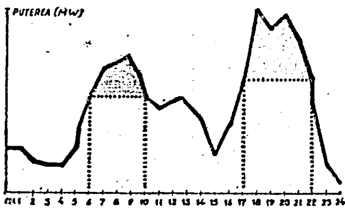
Așa variază consumul de energie electrică în decursul unei zile. Se remarcă faptul că între orele 6-10 dar, mai cu seamă între orele 17-22, puterea absorbită din rețea crește considerabil. Sînt orele în care termocentralele cu funcționare continuă sînt „ajutate” de hidrocentrale. Dar acestea din urmă nu au apă, deci nici putere. Soluția — aplatizarea curbei prin reducerea consumului în aceste ore și deplasarea unor consumuri în zonele în care puterea absorbită e mai mică (orele 13-16 și 22-6).
