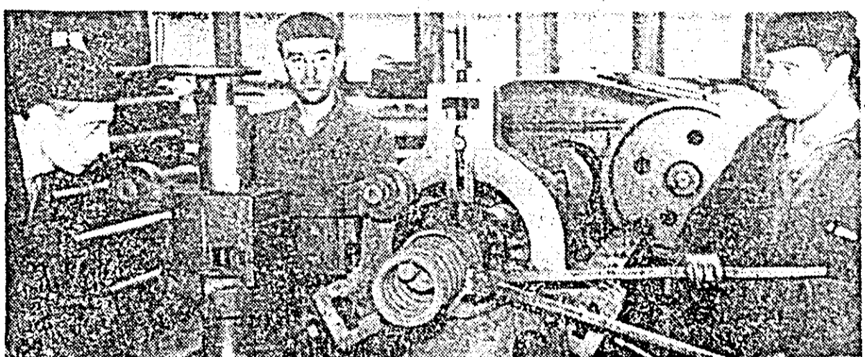
In secția arcuri a Uzinelor de vagoane se duce o hotărîtă bătaie împotriva rebuturilor. Pentru aceasta fiecare operație se execută cu multă atenție. IN FOTOGRAFIE: șeful de echipă Ioan Ilieanu, împreună cu Traian Nadiu și Iosif Ignat efectuînd înfășurarea unui arc.
