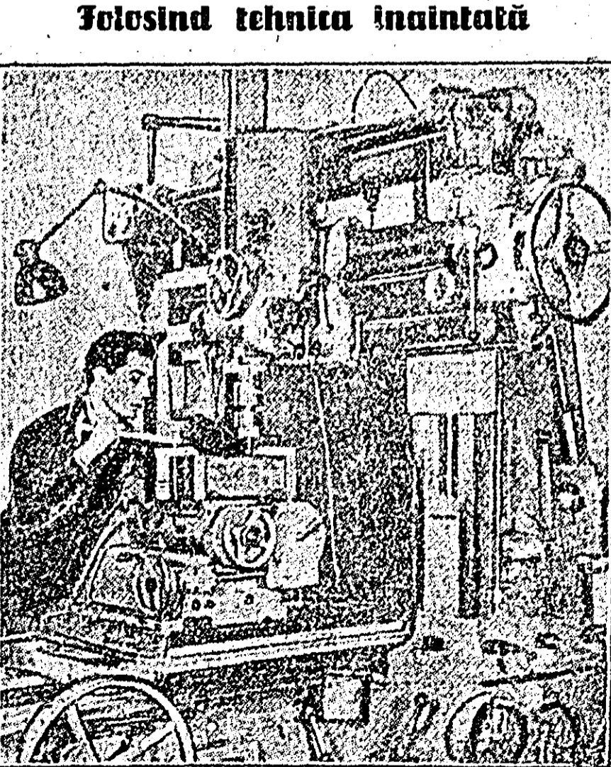
Cu citeva luni în urmă, secția sculărie a uzinelor „Semănătoarea” din capitală a fost înzestrată cu o nouă mașină de înaltă tehnicitate, sosită din R. D. Germană. Este mașina care se vede în clișeu, cu ajutorul căreia se fac operații de alez și găurit prin coordonate. Printr-o deplină utilizare a capacității de lucru a noii mașini, muncitorul Alexandru Vasilescu realizează depășiri medii de normă de 100 la sută.
