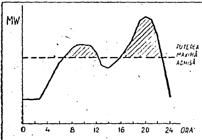
Așa arată (cu linie continuă) curba de sarcină a unei zile normale de lucru în județul Arad. Se observă că peste puterea maximă admisă (linia întreruptă) există două vîrfuri — cel de dimineață și, mai mare, cel de seară. Prin măsurile de limitare a puterilor absorbite din rețeaua de energie electrică, aceste vîrfuri (zonele hașurate) trebuie deplasate în zonele cu consum mai redus (linia continuă și cea întreruptă).
