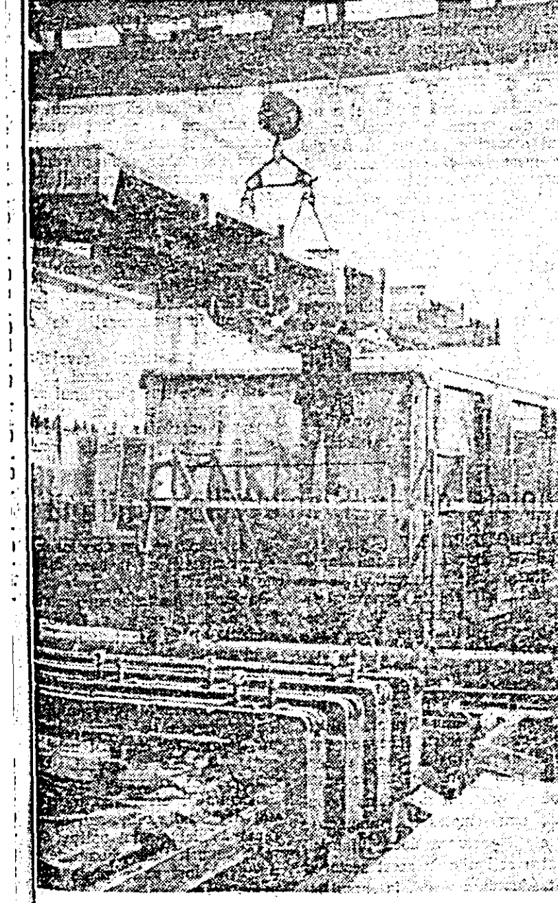
Aspect general din hala de montaj sudură. Se asamblează un nou vagon. El va completa încă un lot care va părăsi uzina.
