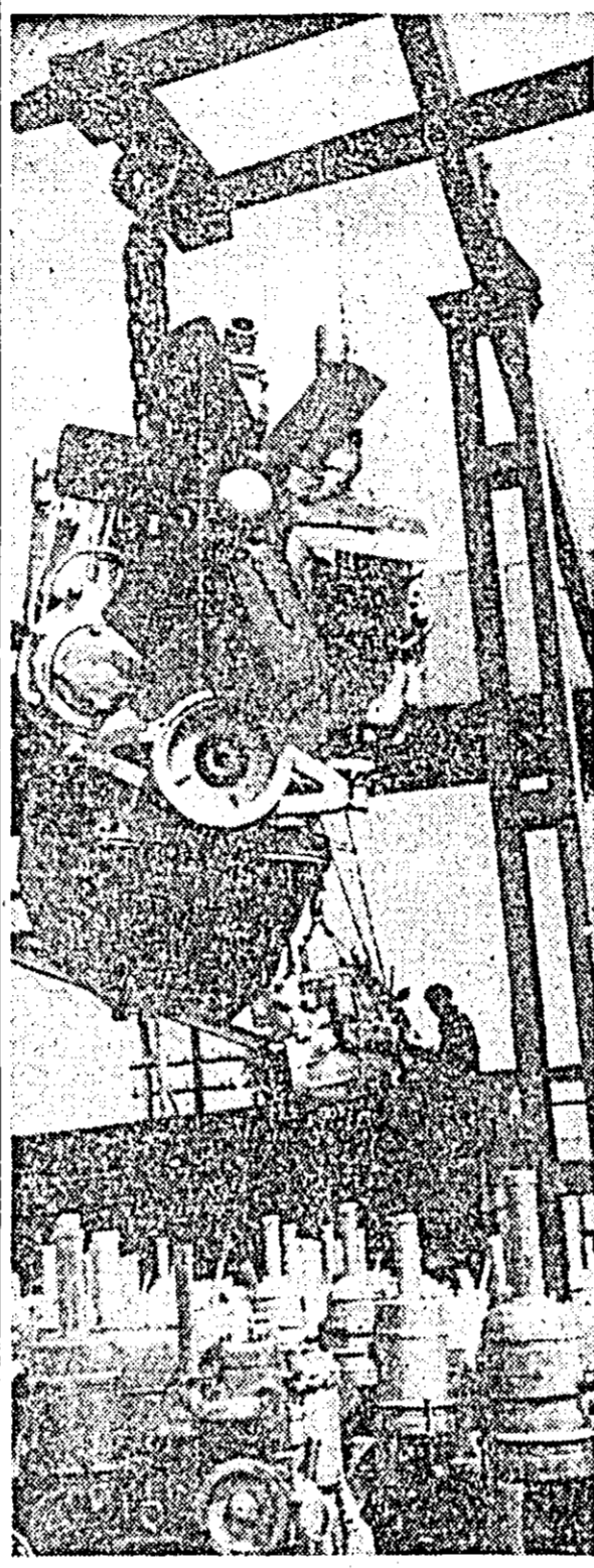
În sectorul IV al Uzinei de reparații din orașul nostru se efectuează un mare volum de reparații la motoarele pentru tractoare.
