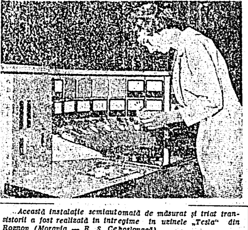
Această instalație semiautomată de măsurat și triat transistorilor a fost realizată în întregime în uzinele „Tesla” din Roznov (Moravia — R. S. Cehoslovaci).
