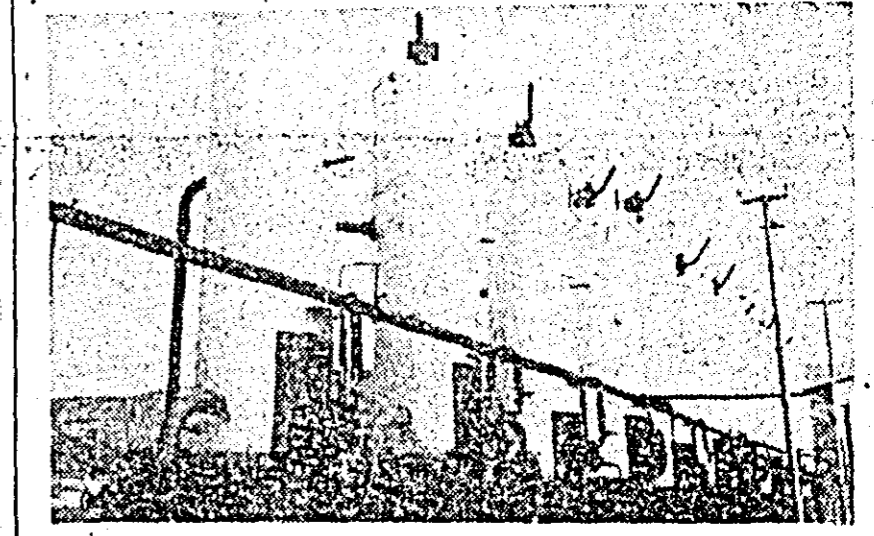
SCHELA DE EXTRACTIE HOLDESTI, JUDEȚUL PRAHOVA. — Aspect din parcul de separatoare al schelei.
