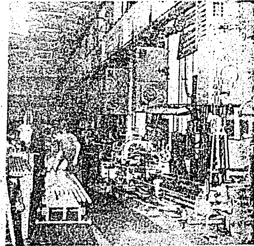
Uzina de strunguri. Vedere generală a liniei de prelucrare a șurubului conductor a axului principal.
