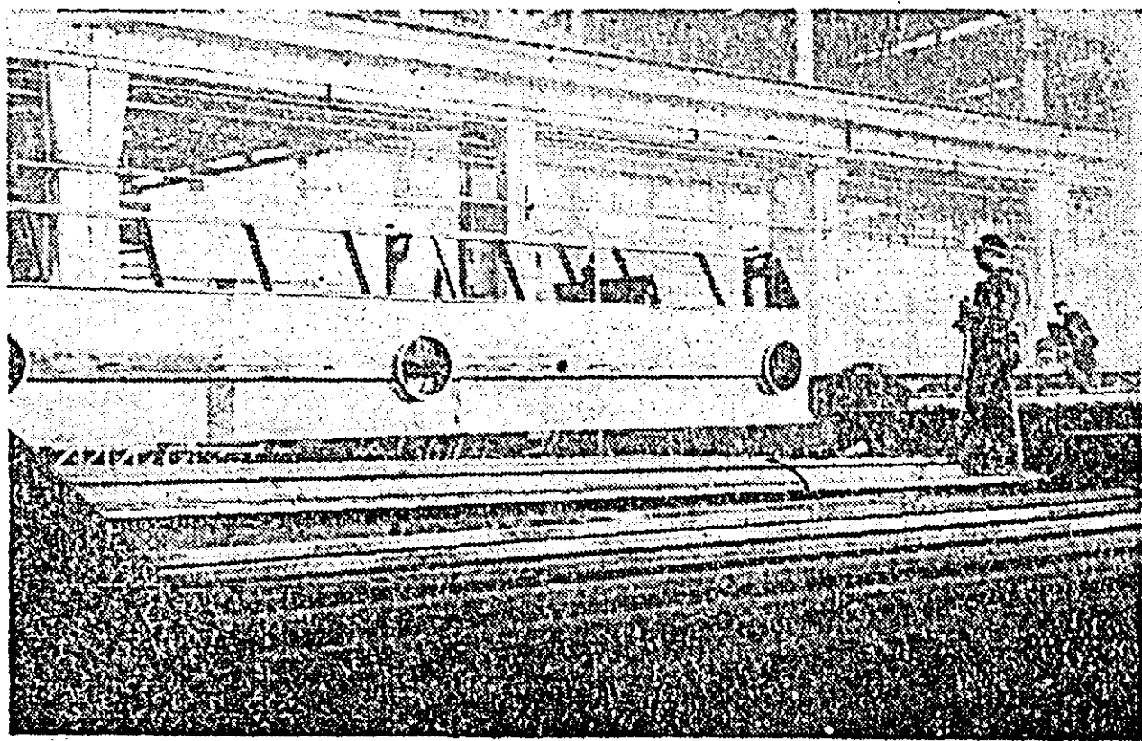
În secția montaj sudură a Uzinelor de vagoane arădene, a cărei imagine v-o prezentăm în clișeu de sus, se asamblează giganticele piese ce compun vagonul. Din această secție vagoanelor pornesc pe fluxul tehnologic spre alte secții care definitivează construcția vagoanelor.
