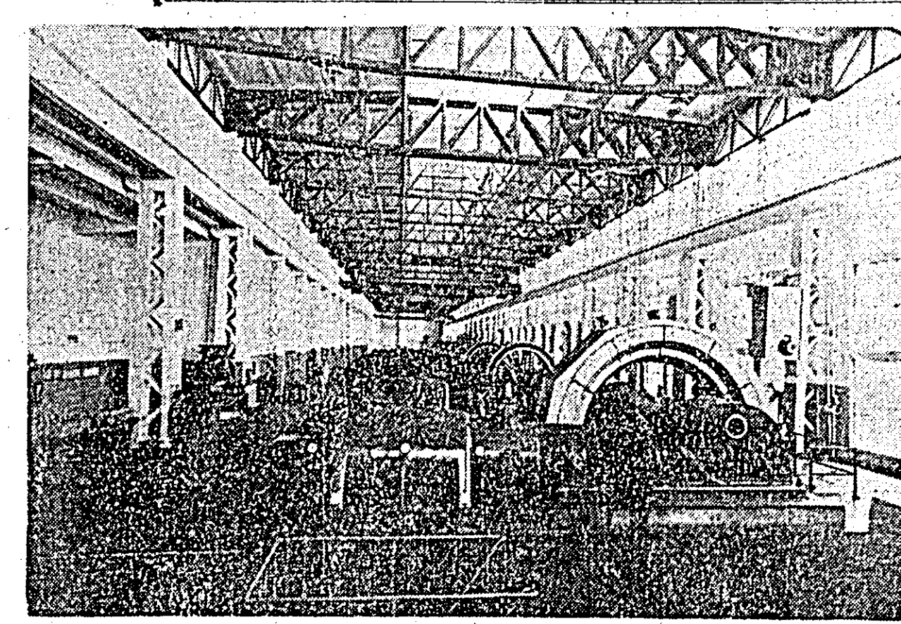
Anul acesta fabrica de azotat de amoniu a Combinatului chimic din Făgăraș va da agriculturii cu 3.000 tone mai multe îngrășăminte față de anul 1962. ÎN FOTO: Fabrica de amoniac — hala de compresoare.
