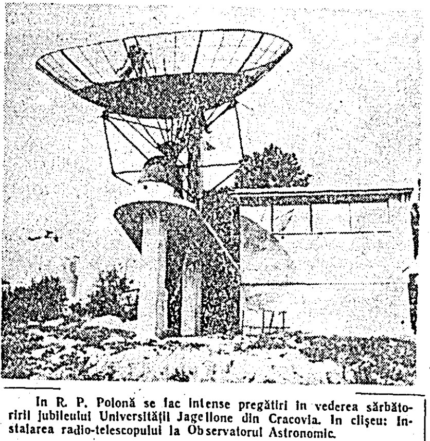
În R. P. Polonă se fac intense pregătiri în vederea sărbătoririi jubileului Universității Jagellone din Cracovia. În clișeu: Instalarea radio-telescopului la Observatorul Astronomic.
