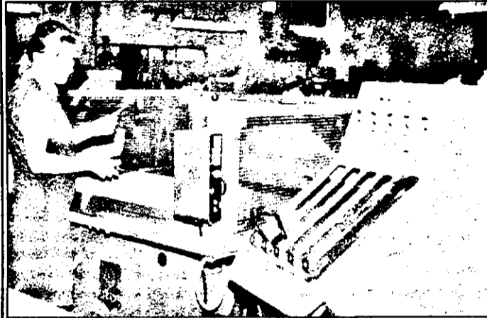
Mașina de croit cu programare, execuție și numărătoare automată a pieselor.
