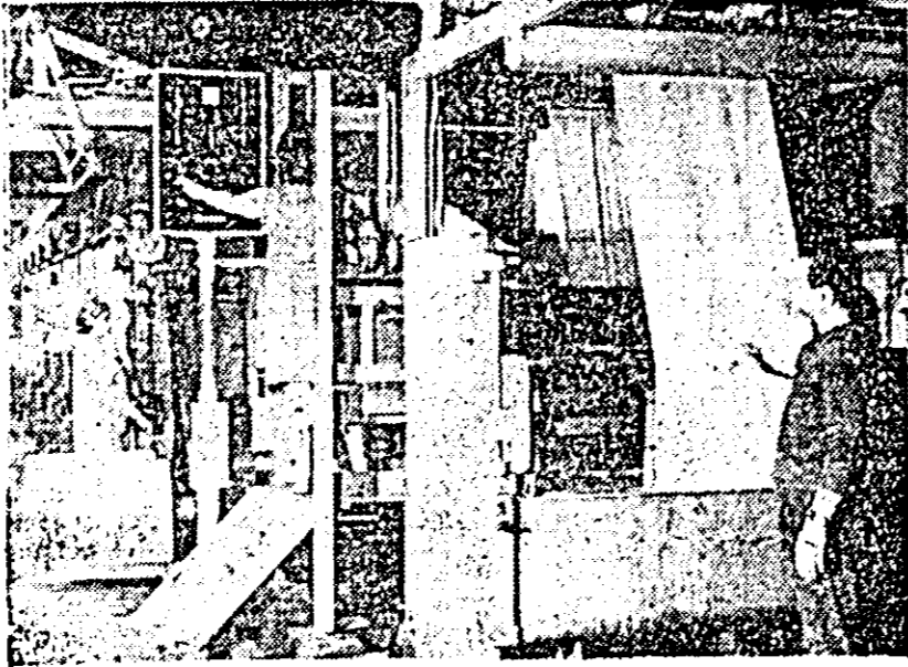
Mașina de apretat pe care o vedeți în cliseul de sus a fost montată de curînd în secția finisaj a fabricii „Teba”. Cu ajutorul ei se pot realiza apreturi superioare, neșfonabile și o productivitate mărită (16.000 m.l. în opt ore).
