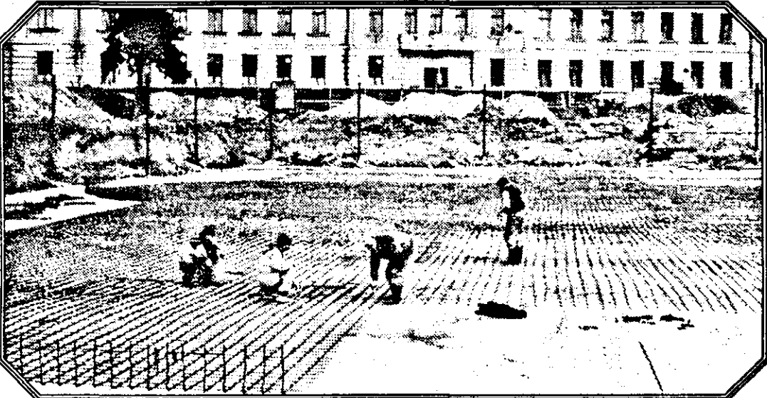
Șantierul Catedralei Ortodoxe Arad: se lucrează la armarea radierului general (montarea plasei de jos). Conturul viitoarei Catedrale este pus, deja, în evidență. Foto: VIOREL MUSCA
