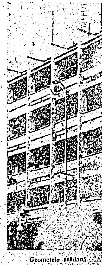
Geometrie arădani
