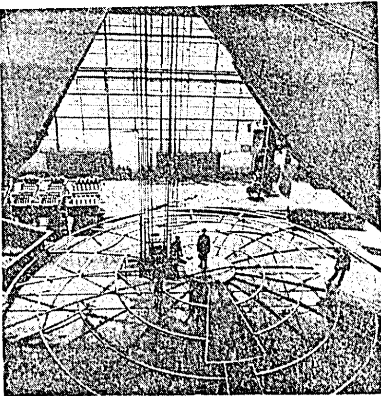
În secția cazangerie a uzinelor „Grivița Roșie” din Capitală se confecționează un rezervor de mari proporții destinat uzinei de aluminiu de la Slatina.
