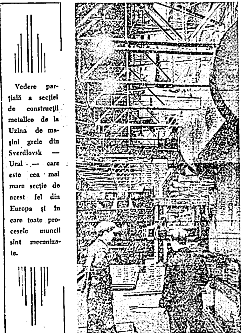
Vedere parțială a secției de construcții metalice de la Uzina de mașini grele din Sverdlovsk — Ural — care este cea mai mare secție de acest fel din Europa și în care toate procesele muncii sînt mecanizate.
