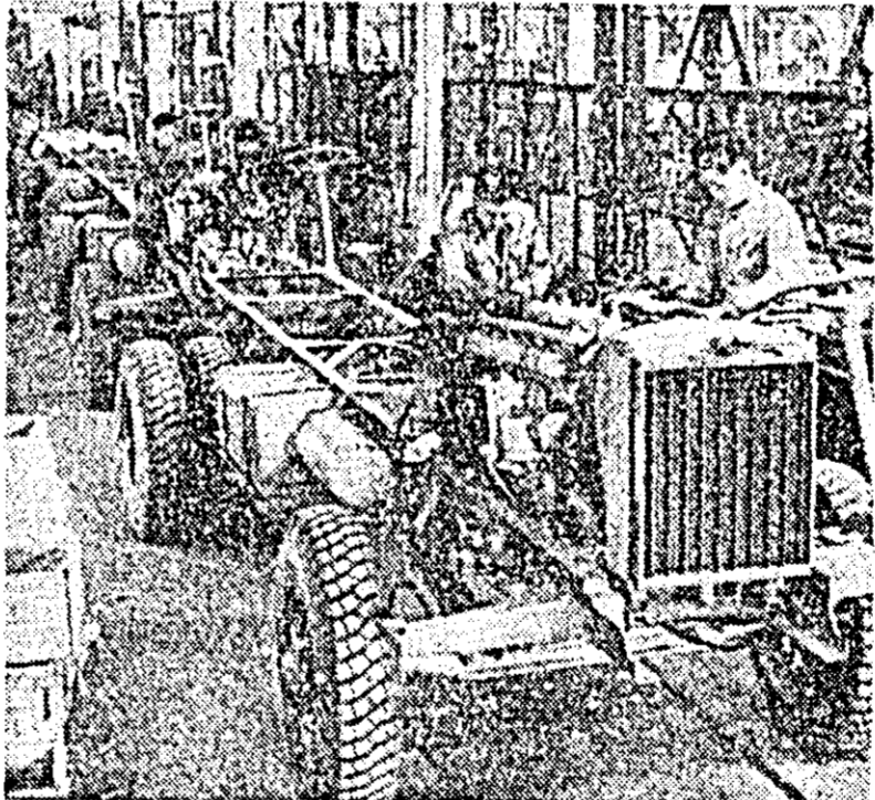
Aspect de muncă în secția de asamblare a Uzinei de automobile din Tșinan: se asamblază autocamioane „Yellow River”. (R. P. Chineză).
