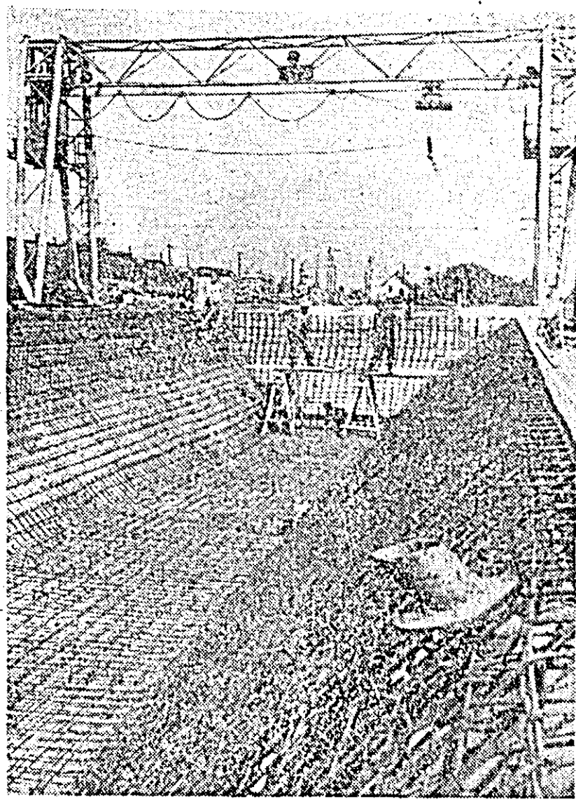
La fabrica „Libertatea” se lucrează în acest zilo la un bazin destinat conservării lemnului. Prin aceasta se va evita uscarea excesivă a lemnului folosit la confecționarea calapoadelor.
