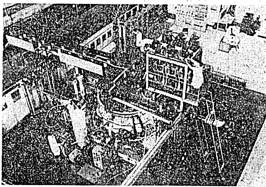
U.R.S.S. — Obținerea plasmelor termonucleare fierbinți prin încălzirea hidrogenului greu pînă la temperaturi solare, izolarea unui astfel de plasmă de pereții reactorului — iată problemele care se rezolvă la instalațiile de cercetări de tipul Tokamak, create de Institutul de energie atomică „L. V. Kurceatov”. În CLIȘEU: Vederea generală a instalației Tokamak 3.
