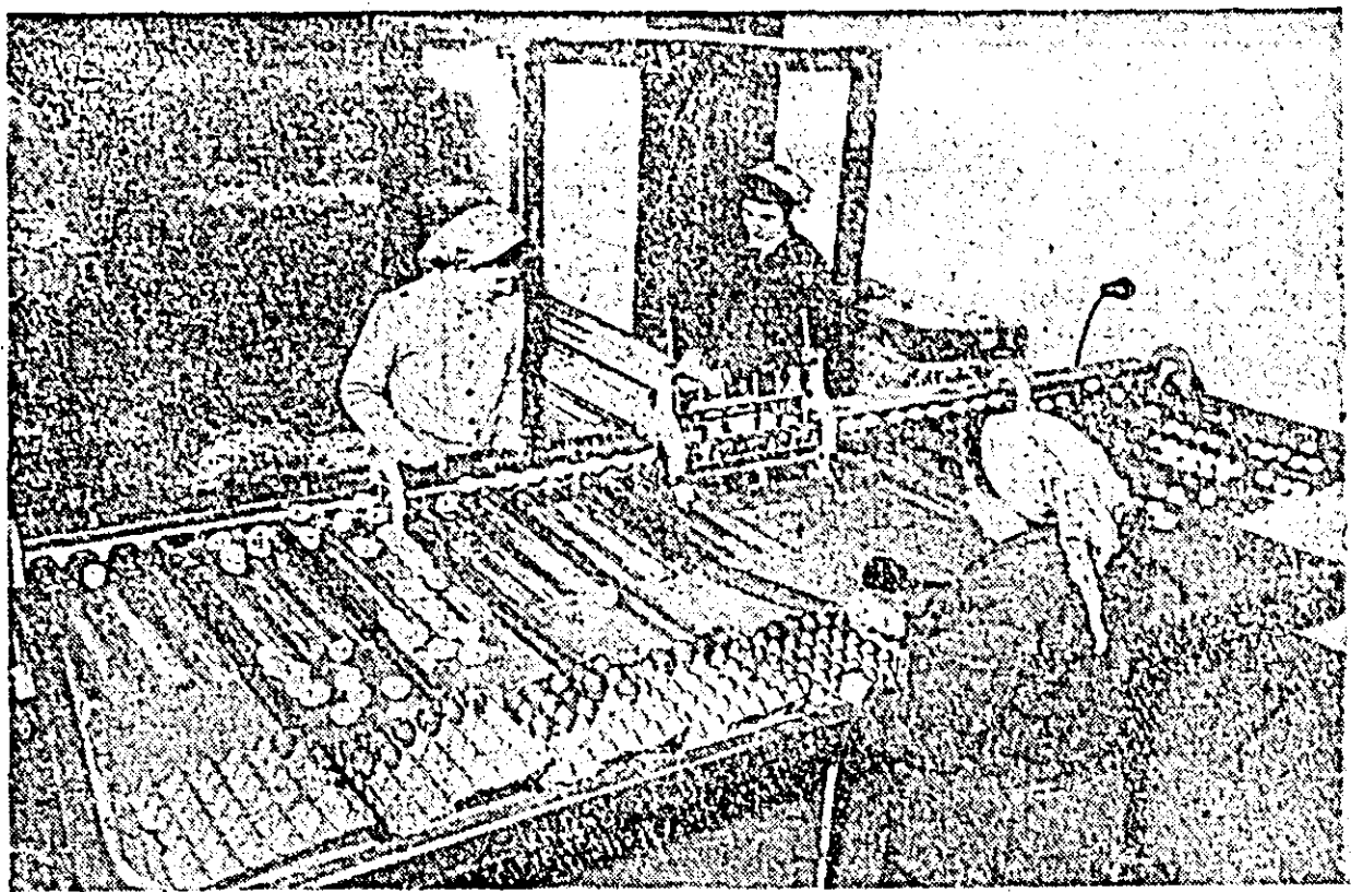
La stațiunea de incubație a IRAVICOP Arad funcționează și o mașină de sortat ouă. Iată în clipă această mașină în lucru, sortînd ouăle după greutate.
