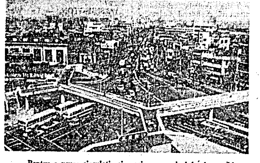
Pentru a ușura circulația și a micșora pericolul de accidente, autoritățile din Tokio au hotărît construirea unui drum suspendat într-un loc de mare trafic (60.000 vehicule zilnic) — stația Shinjuku. Lucrările au început în decembrie anul trecut, fiind terminate după șase luni.
