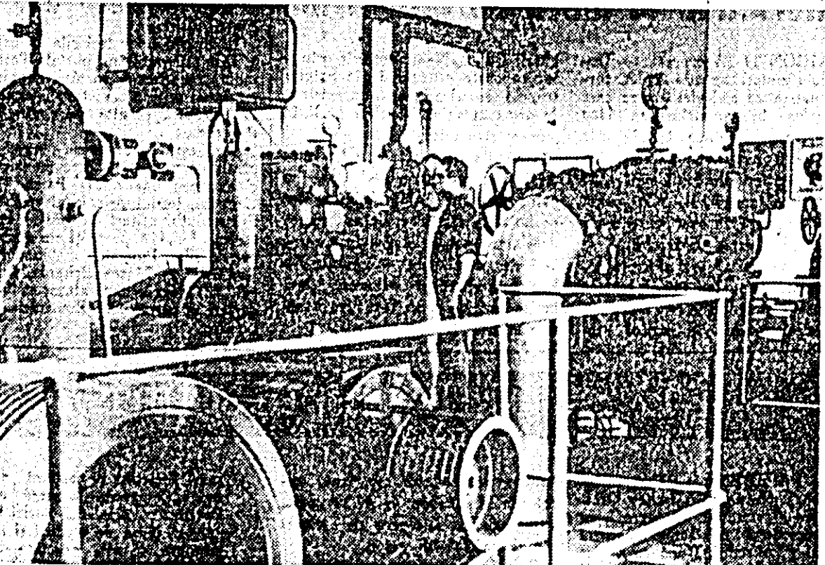
Sala compresoarelor de la Antrepozitului Frigorifer. 6 agregate întrețin în camerele de depozitare temperaturi între — 16 și — 22° C — iar în tunelurile de congelare pînă la — 35° C. O adevărată iarnă.
